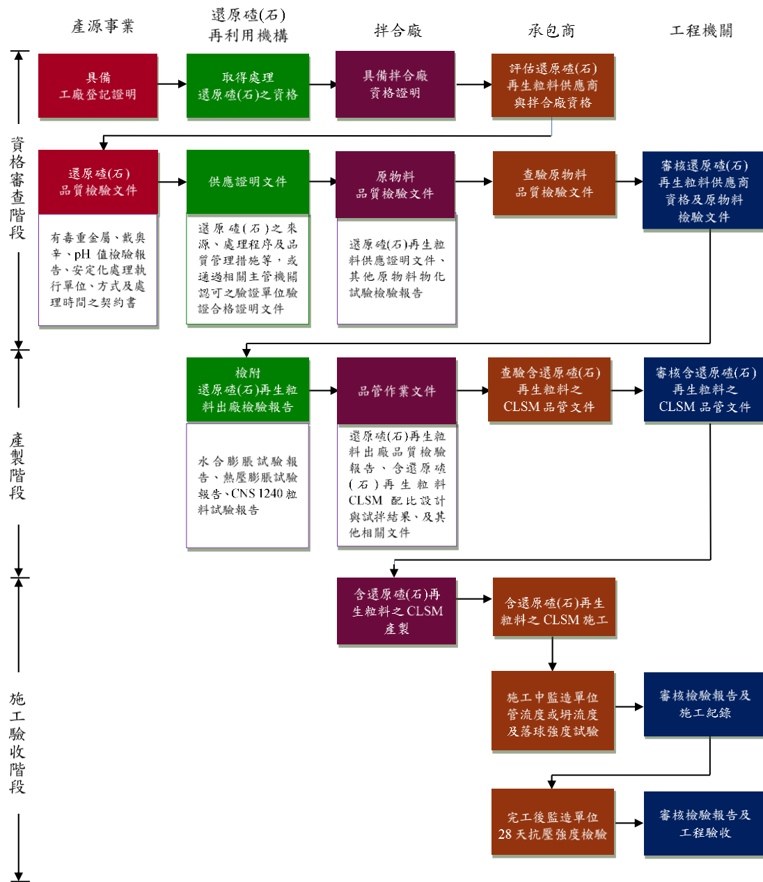
圖 7-1 含還原渣(石)CLSM 品管作業流程
